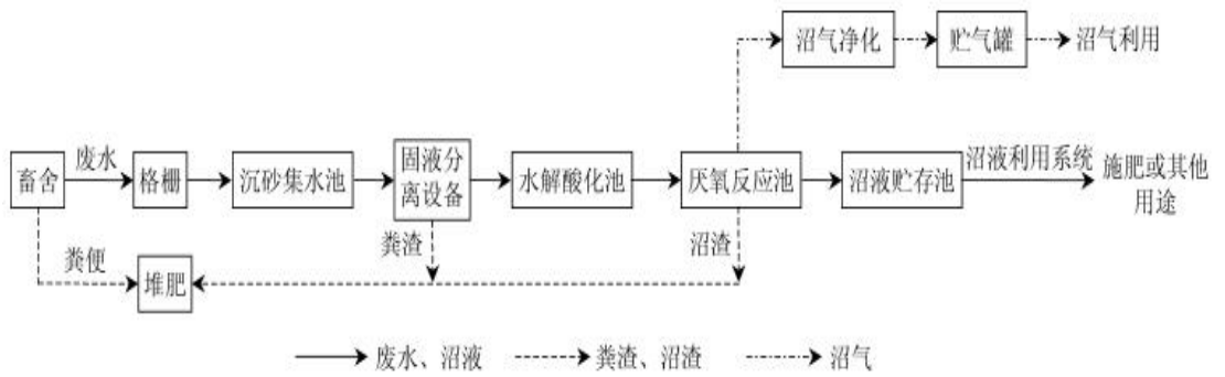
图 2.2-5 模式Ⅱ工艺基本流程
