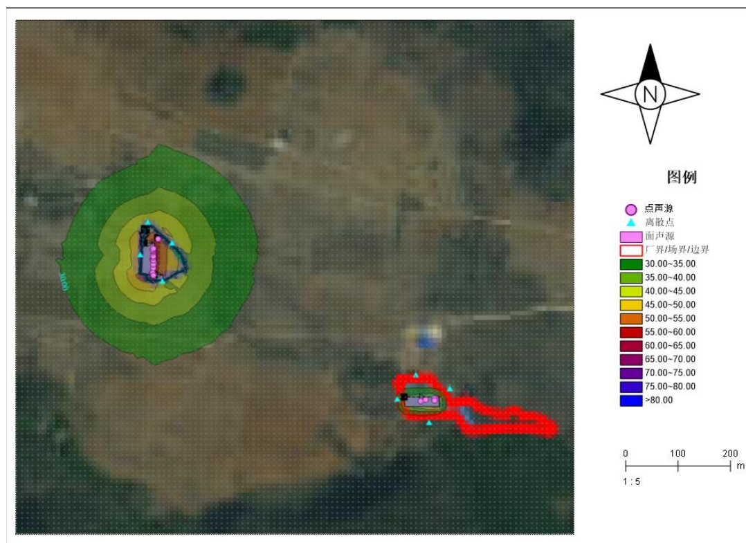
图 4.2-5 采取措施后项目噪声等声值线图
