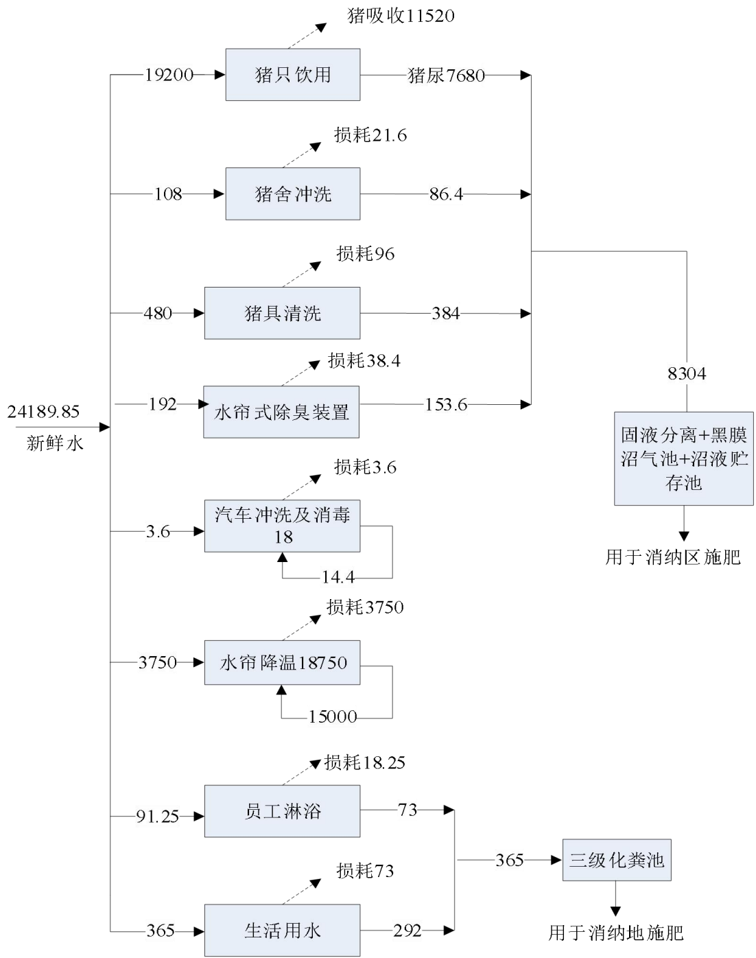
图 2.3-7 扩建项目水平衡图 单位：m³/a
