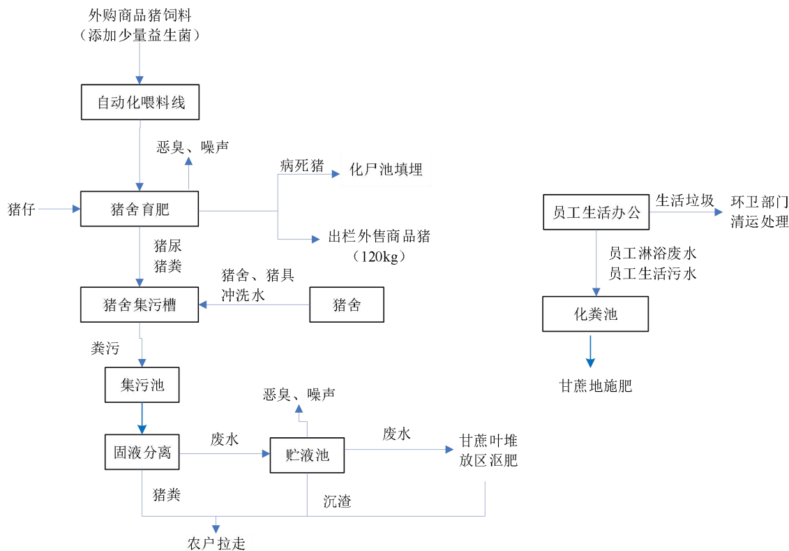
图 2.1.5-1 现有工程养殖过程及产污环节示意图
