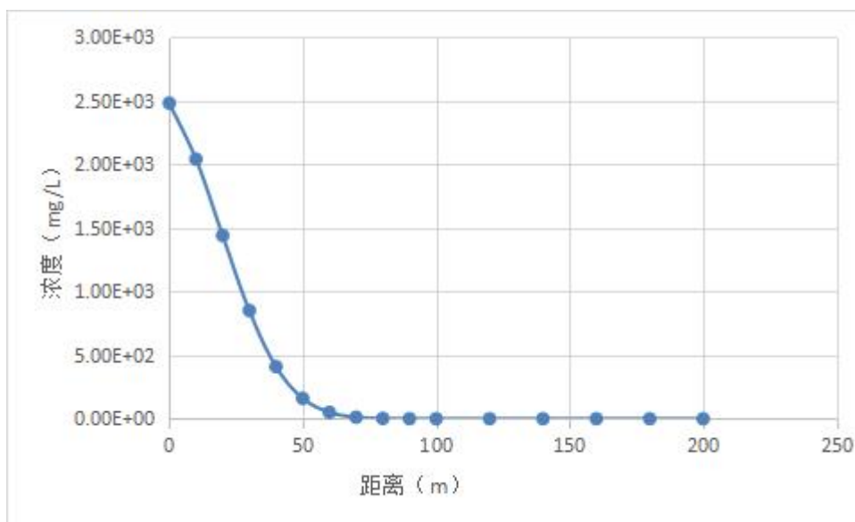
图4.2.3-1 集污池COD Mn 泄漏100天，COD Mn 污染扩散距离图
