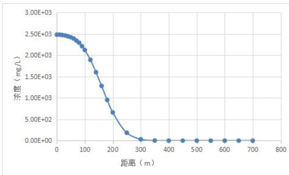
图4.2.3-2 集污池 \text{COD}_{\text{Mn}} 泄漏1000天, \text{COD}_{\text{Mn}} 污染扩散距离图
