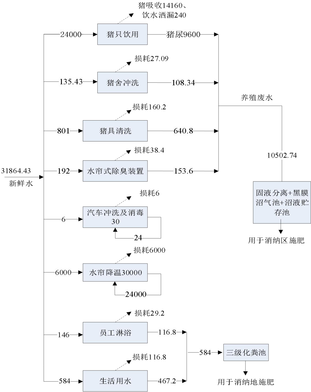
图 2.3-8 扩建后全厂水平衡图 单位： \text{m}^3/\text{a}
