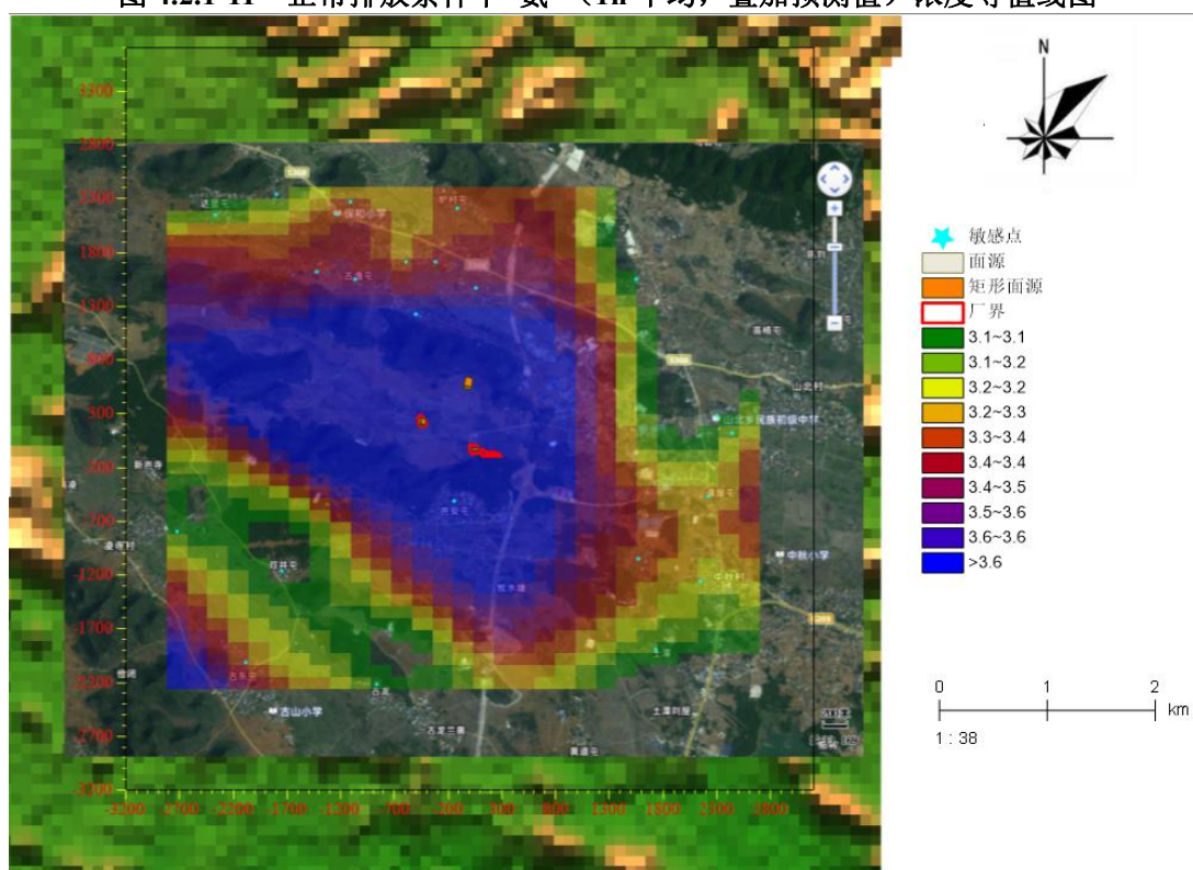
图 4.2.1-13 正常排放条件下硫化氢（1h 平均，叠加预测值）浓度等值线图
