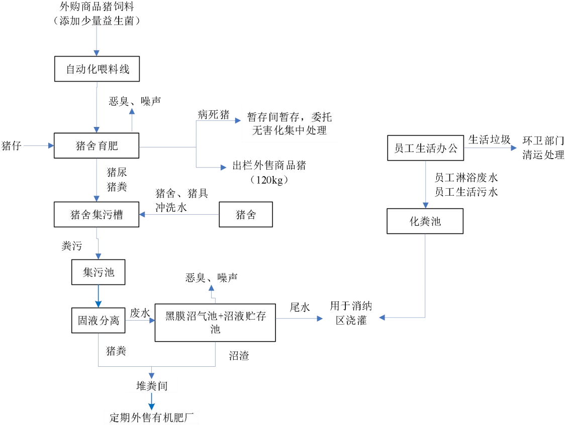
图 2.3-6 项目养殖过程及产污环节示意图
