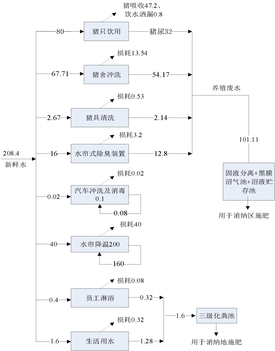
图 2.3-9 扩建后全厂水平衡图 单位：m³/d
