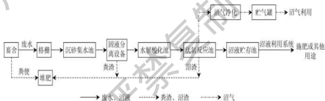
图 2.2-3 模式II工艺基本流程
