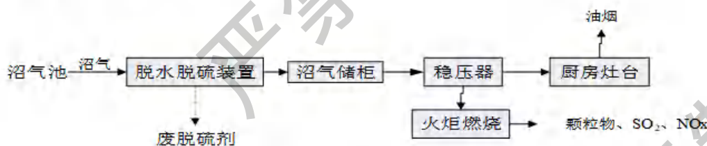
图 2.2-5 沼气工程工艺流程图
