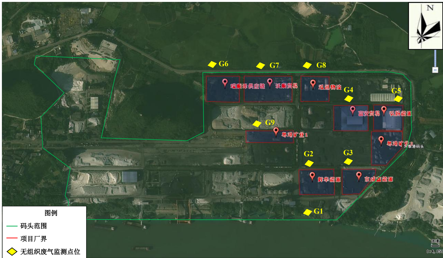
附图 3 项目无组织排放废气监测布点示意图（本项目厂界无组织废气监测点位为下图中的 G1、G4，验收期间主导风向为南风）
