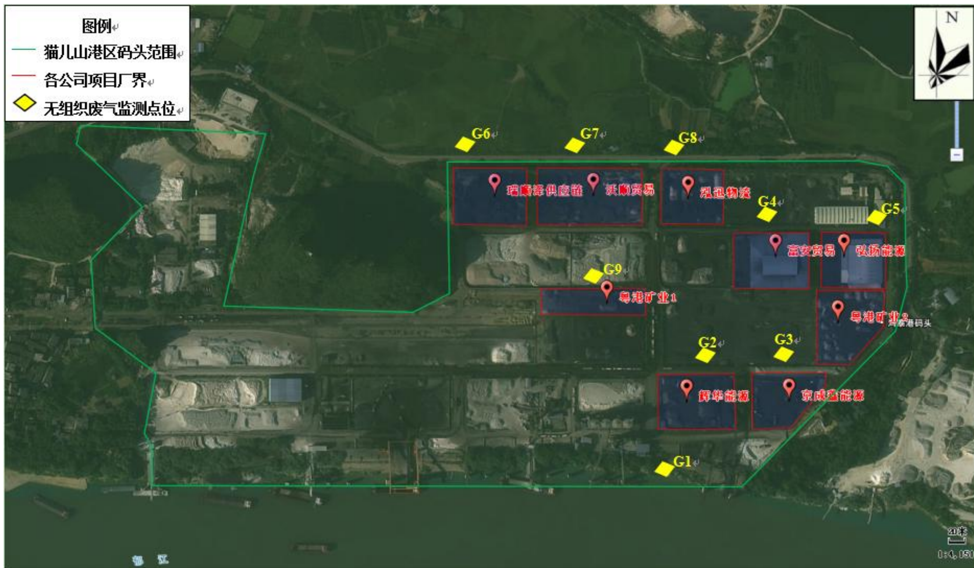
附图 3 项目无组织排放废气监测布点示意图（本项目厂界无组织废气监测点位为下图中的 G1、G5 和 G9，验收期间主导风向为南风）
