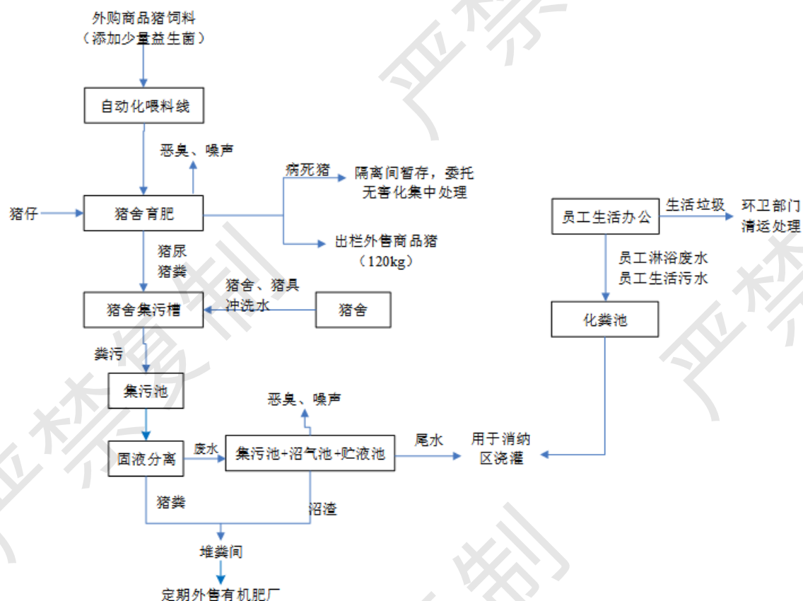
图 2.2-6 项目生产过程及产污环节示意图
