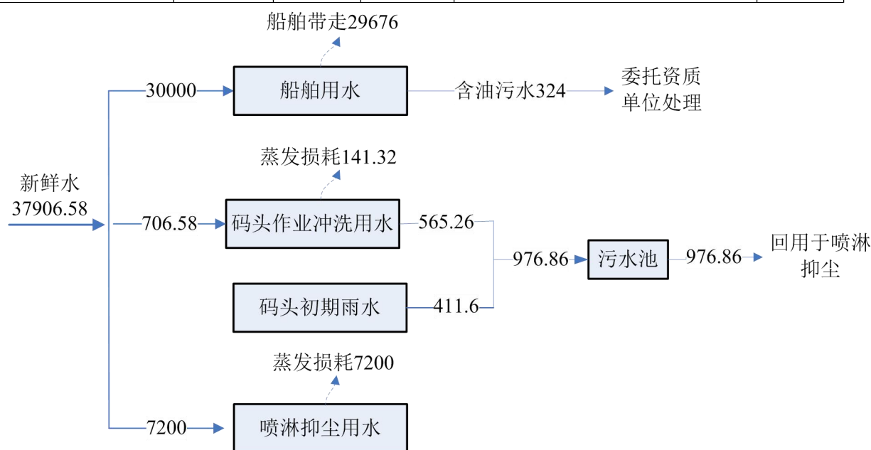
图 2.3-1 本工程水平衡图单位：m 3 /a
