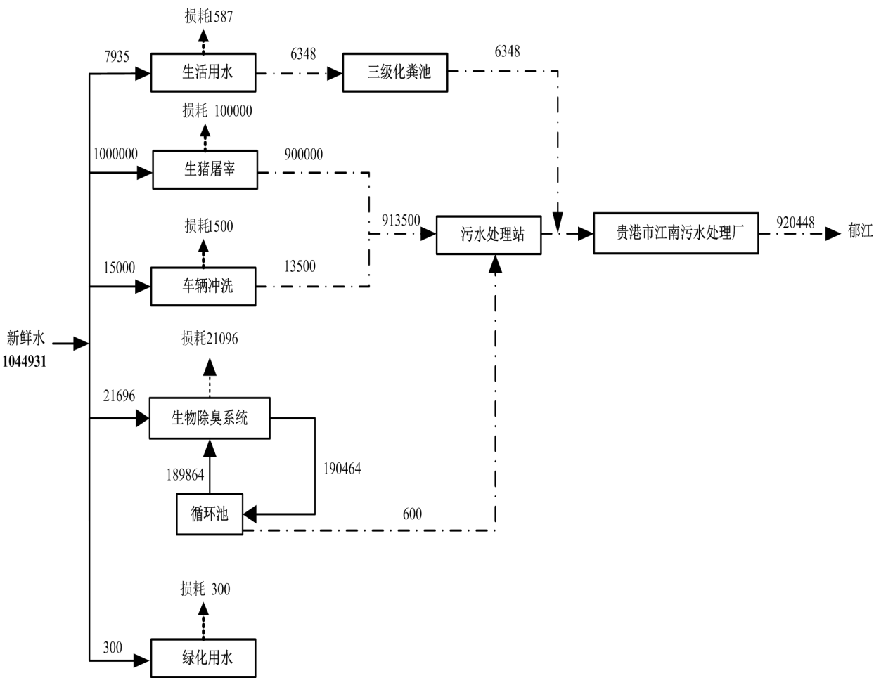
图 2.3-5 项目变更后水平衡图 单位：m³/a
