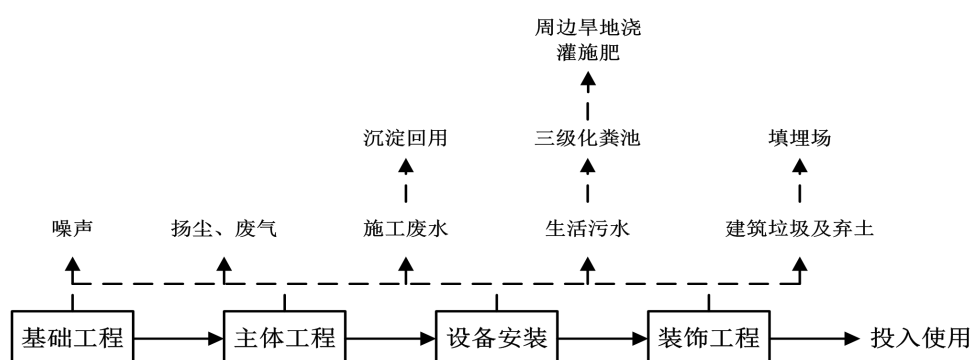
图2.3-1 施工期工艺流程及产污环节分析图
