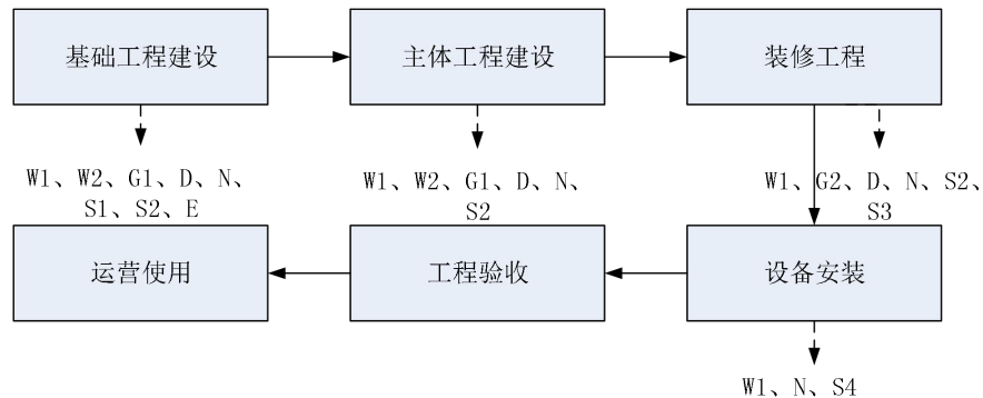
图 2.2-1 项目施工工艺及产污节点图
