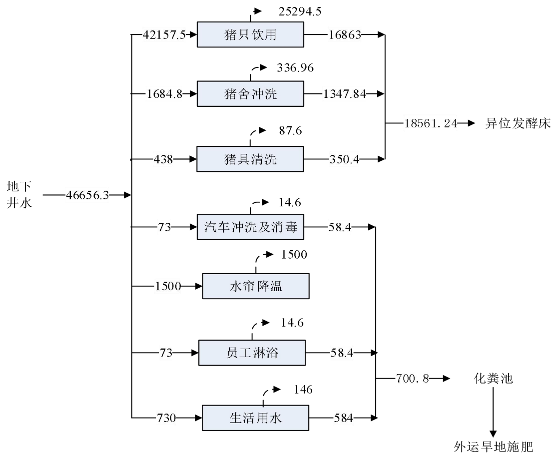
图 2.2-8 项目水平衡图 单位：m³/a
