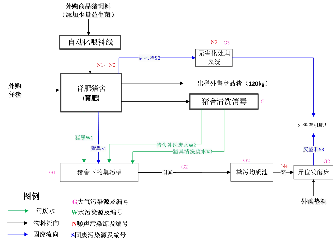
图 2.2-7 项目生产过程及产物环节示意图
