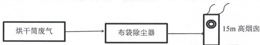
图2 烘干筒废气处理工艺及其监测点位
