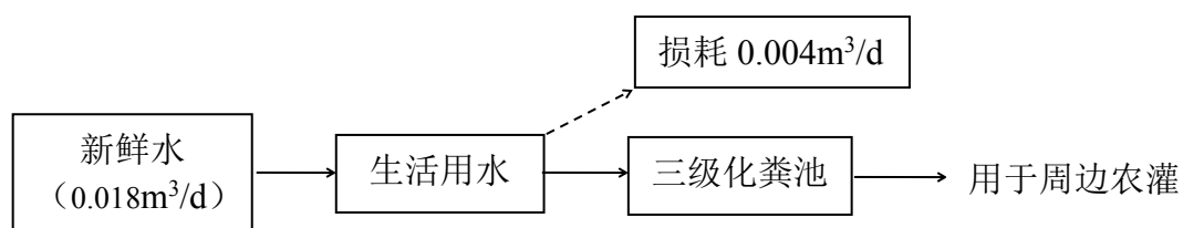
图 2-1 厂区用水平衡图 m³/d
