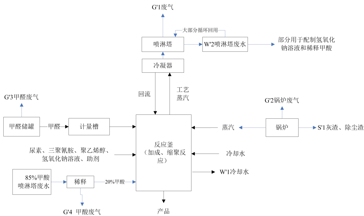
图 2.1-3 环保胶水生产工艺流程及产污环节图（注：各设备均产生噪声）
