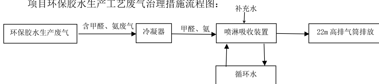
图 5.1-1 项目环保胶水生产线废气污染防治措施图
