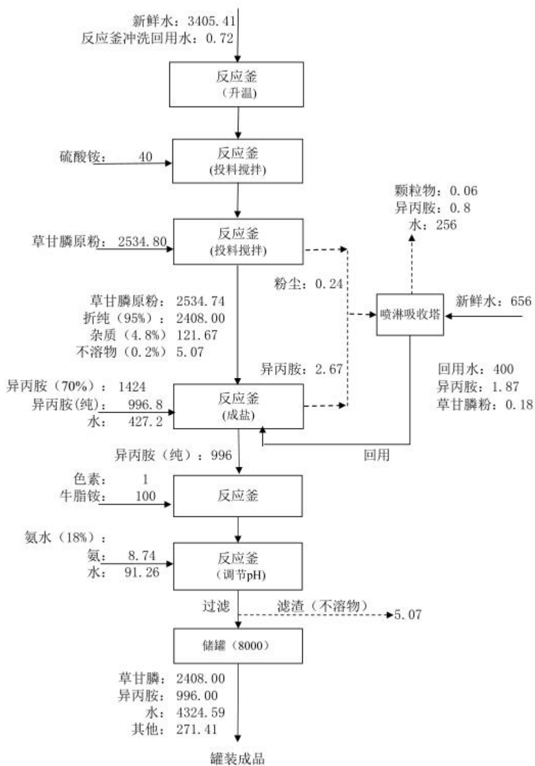
图 2.1-4 项目全年生产物料平衡图 t/a
