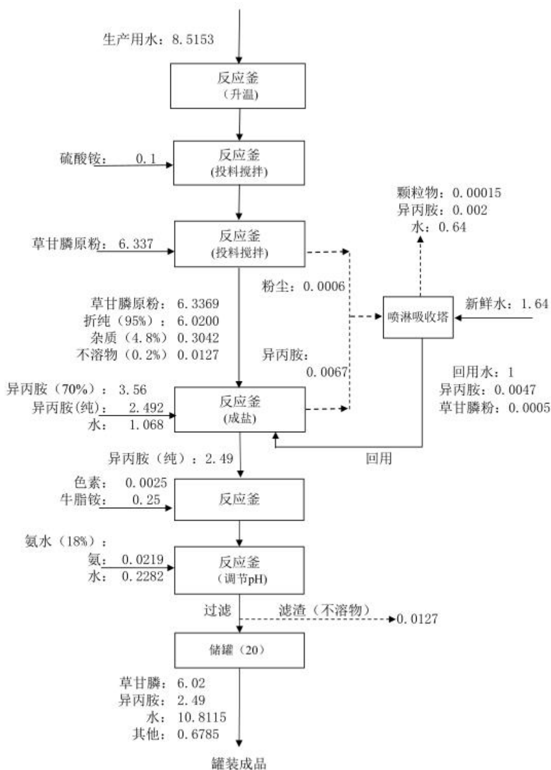
图 2.1-4 项目单个反应釜生产物料平衡图 t/釜·批次
