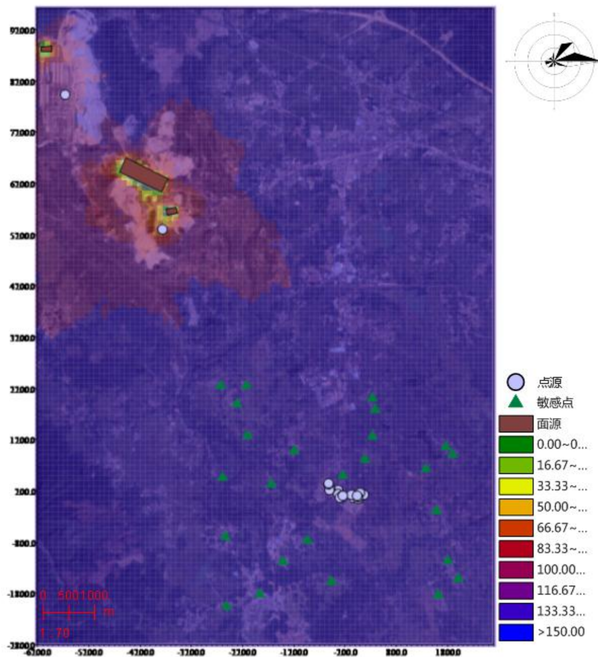
图 4.2.1-10 正常排放条件下 PM 10 日均浓度等级线图（保证率 95%，已叠加背景值）
