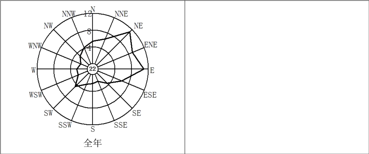
图 4.2.1-1 平南县四季和年风向玫瑰图（1998-2017 年）
