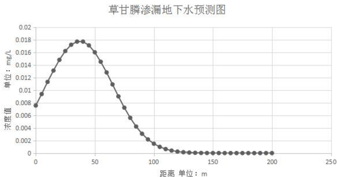
图 4.2-1 泄漏第 100 天，草甘膦污染扩散距离图
