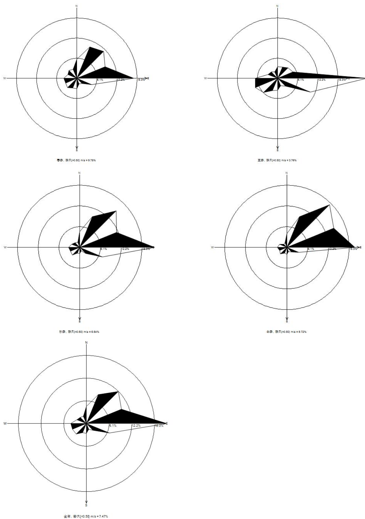
图 4.2.1-5 平南县 2017 年风玫瑰图
