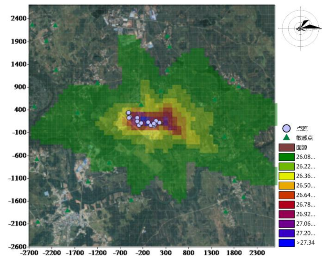
图 4.2.1-6 正常排放条件下二氧化硫日均浓度等级线图（保证率 98%，已叠加背景值）
