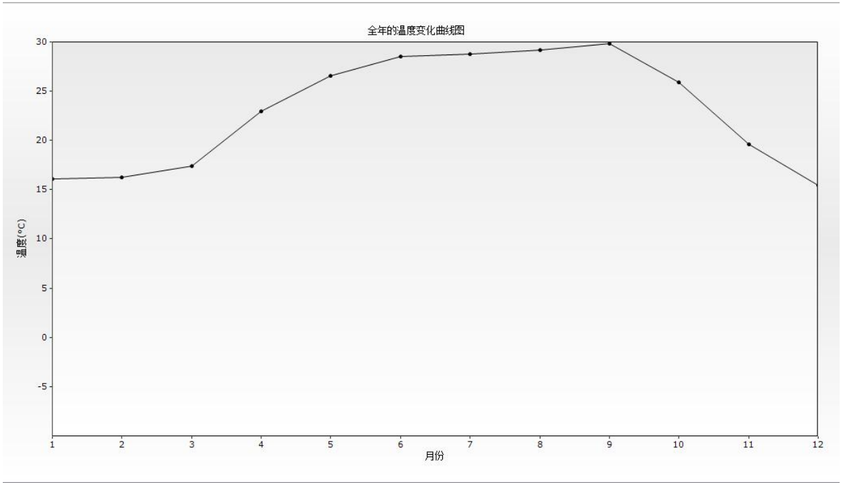
图 4.2.1-2 2017 年平均温度的月变化曲线图
