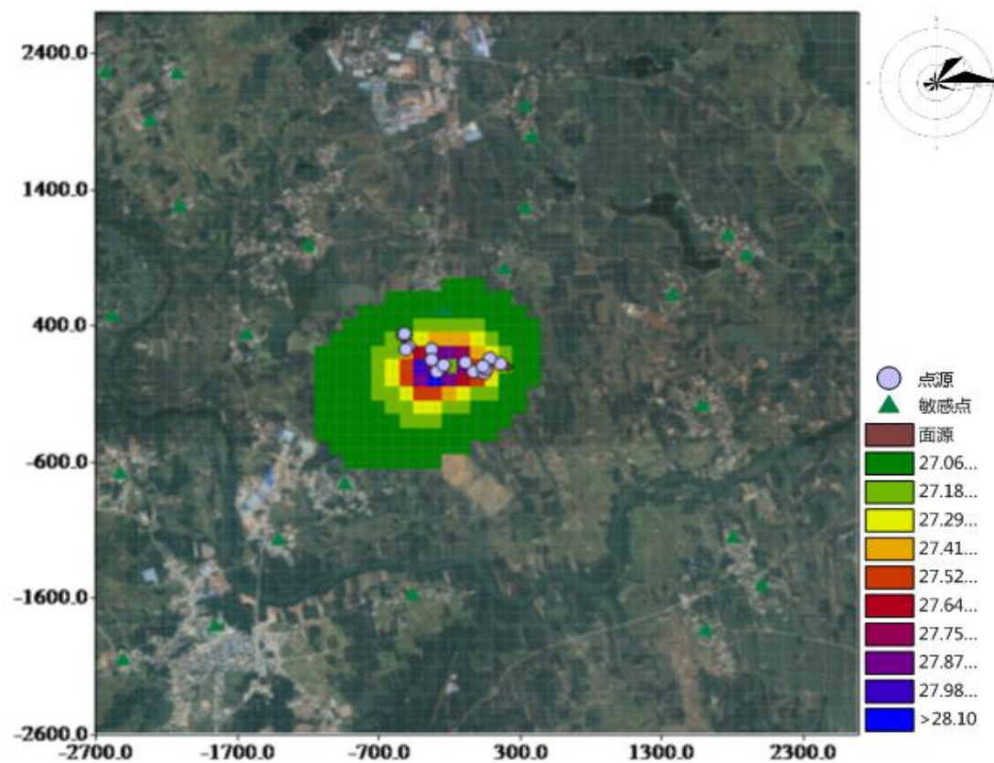
图 4.2.1-9 正常排放条件下二氧化氮年均浓度等级线图（已叠加背景值）
