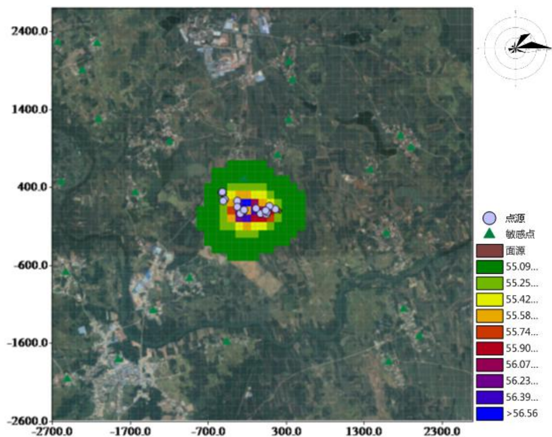
图 4.2.1-8 正常排放条件下二氧化氮日均浓度等级线图（保证率 98%，已叠加背景值）
