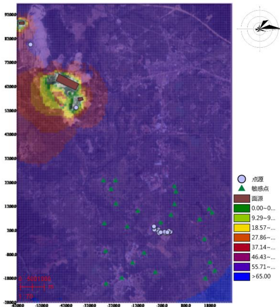
图 4.2.1-11 正常排放条件下 PM 10 年均浓度等级线图（已叠加背景值）
