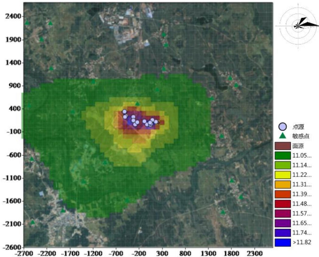
图 4.2.1-7 正常排放条件下二氧化硫年均浓度等级线图（已叠加背景值）
