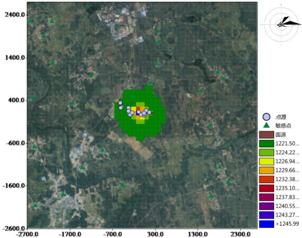
图 4.2.1-12 正常排放条件下非甲烷总烃 1h 平均浓度等级线图（已叠加背景值）
