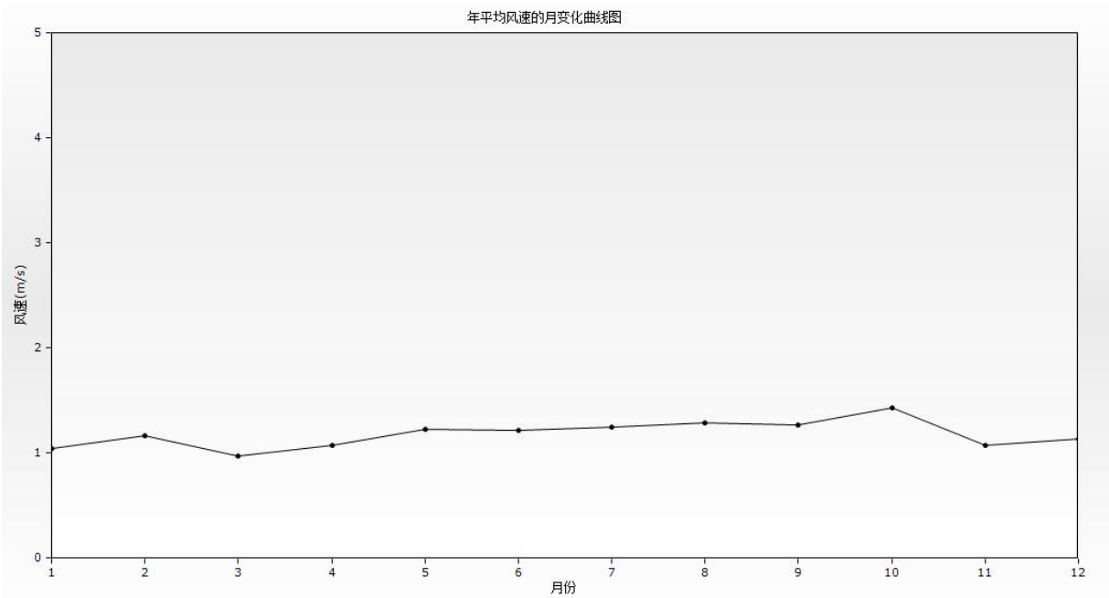
图 4.2.1-3 2017 年月平均风速变化情况图
