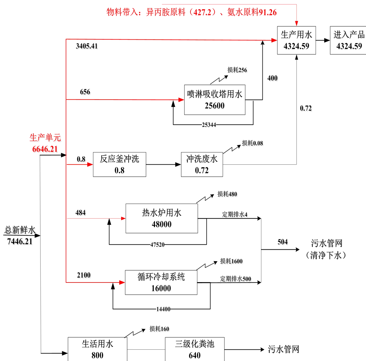
图2.1-5 建设项目运营期水平衡图 (m 3 /a)
