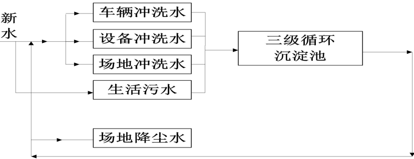
图 3-2 生产废水处理流程示意图
