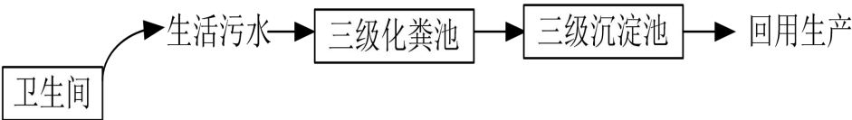
图 3-3 生活污水处理流程示意图
