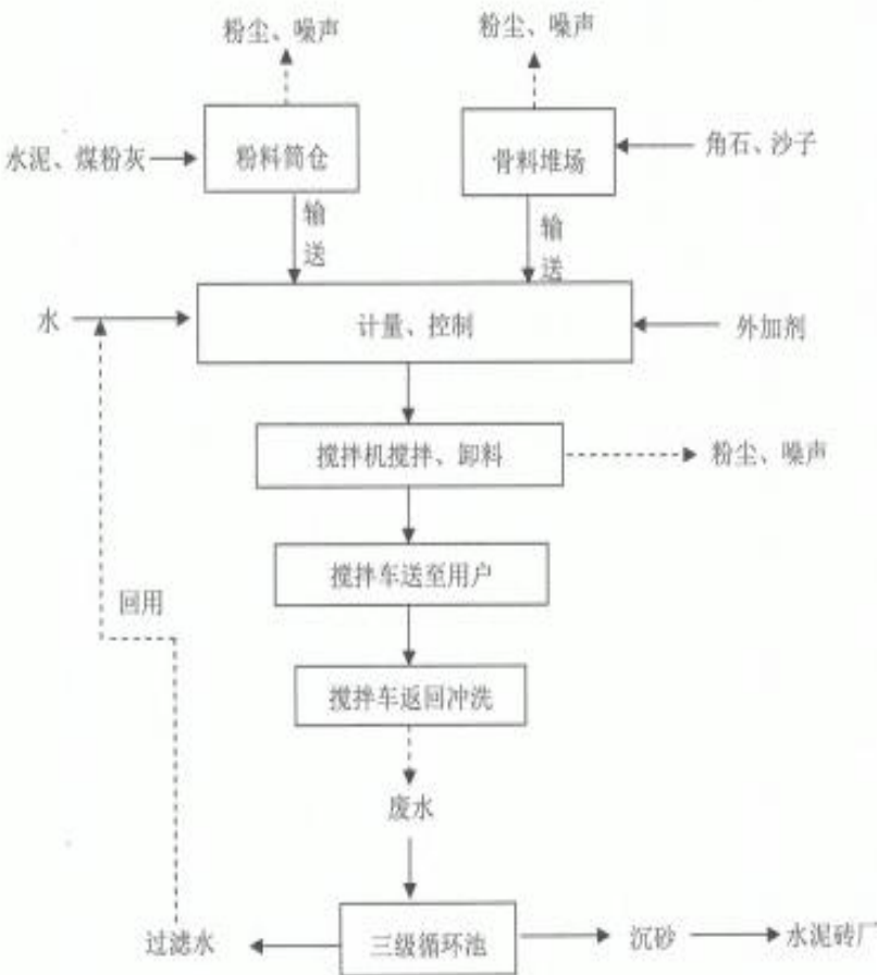
图 1 生产工艺及产污环节示意图
