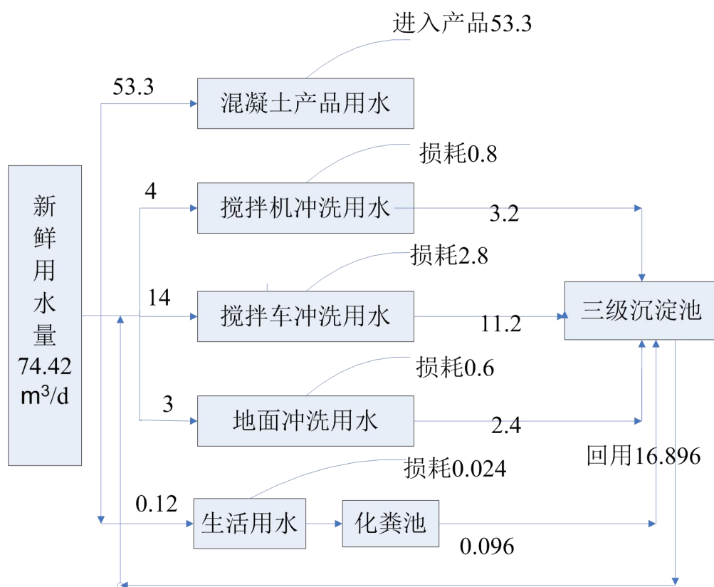
图2-1 项目日水平衡图 (m³/d)
