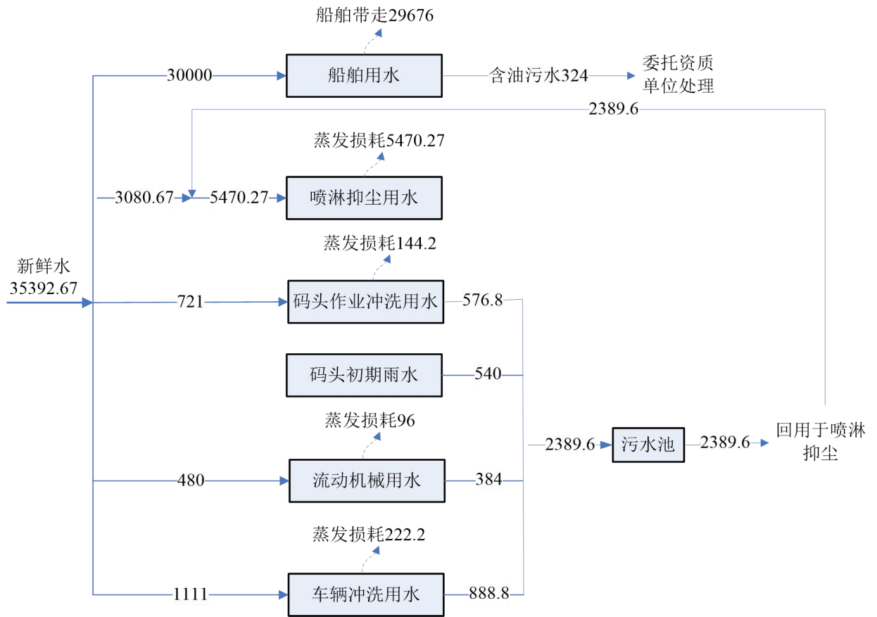
图 2.3-1 本工程水平衡图单位: m³/a
